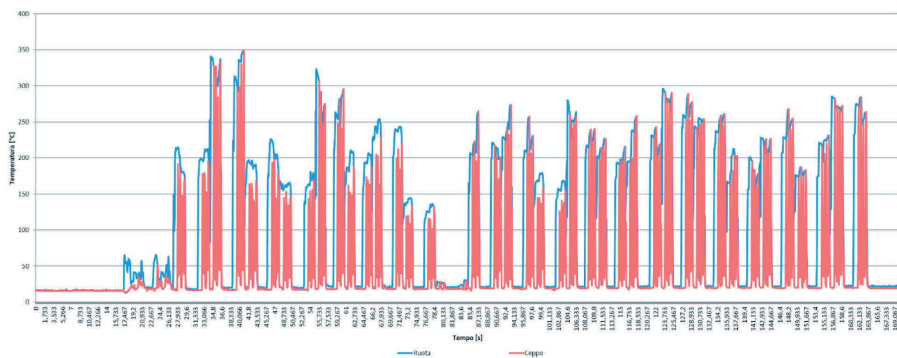
Figura 4 – Andamento delle temperature dell'impianto frenante (ruota e ceppo) per il treno INRAIL prova 2. Figure 4 – Temperature development of the braking system (wheel and brake block) for the INRAIL train test 2.
