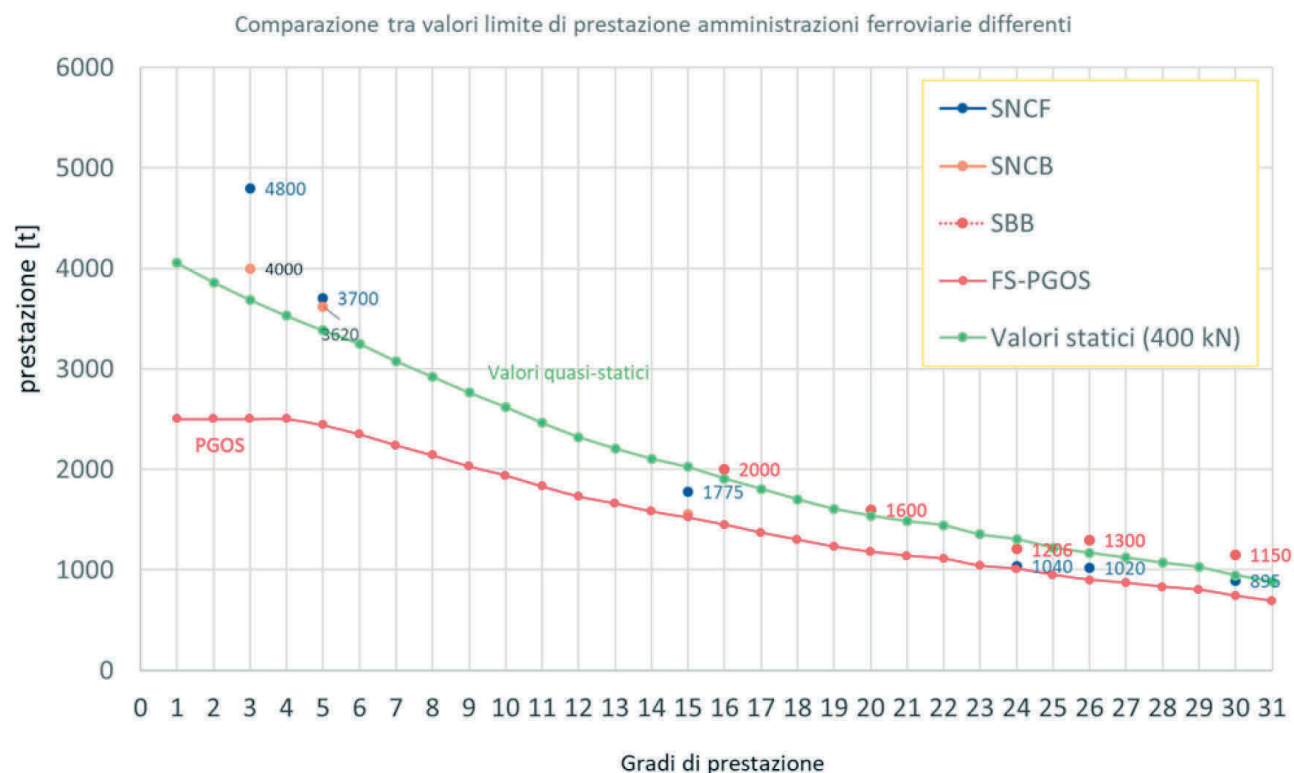
Figura 1 – Comparazione tra gradi di prestazione e massa rimorchiabile in tonnellate includendo i risultati di calcolo in condizioni quasi-statiche riferiti ad uno sforzo al gancio di 400 kN.
